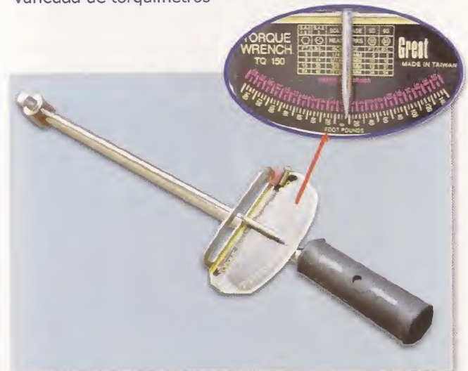
Torquímetro por puntos
